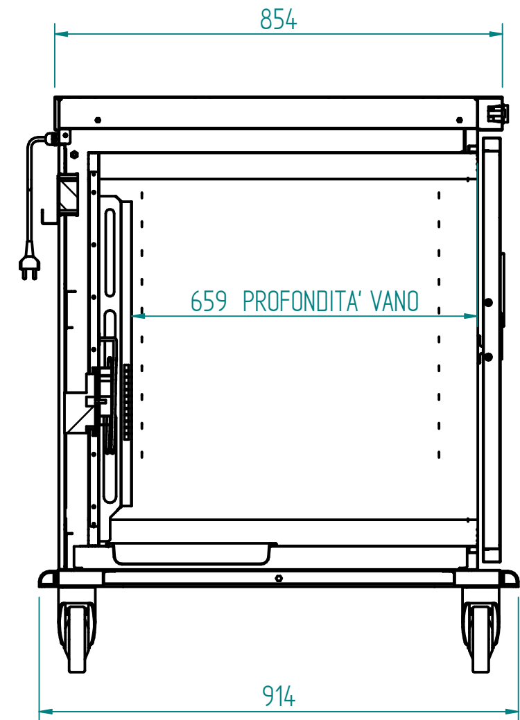
SEZIONE A-A
